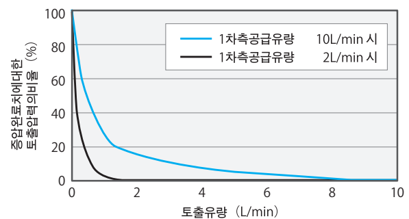
AU2531-0□/AU2530-0M□ 2차측토출유량특성도
