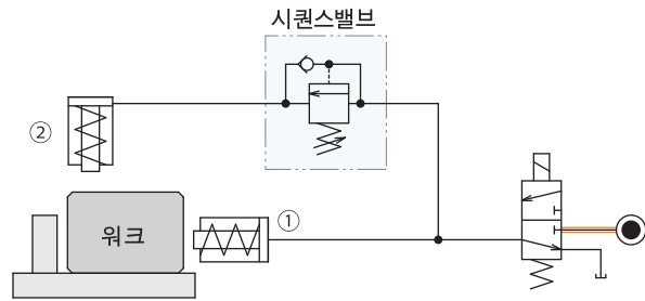
회로도
