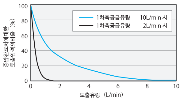
AU2521-0□/AU2520-0M□ 2차측토출유량특성도
