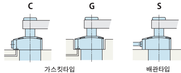
가스킷타입
