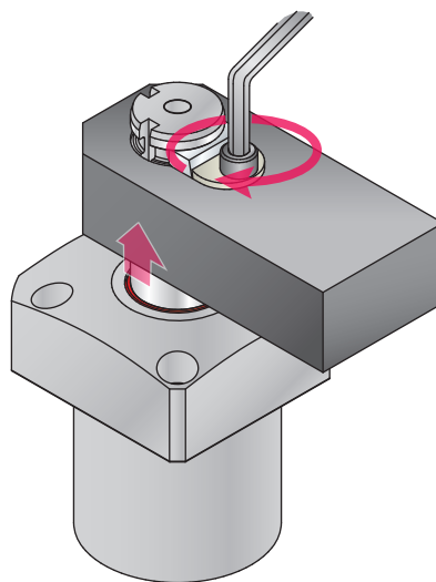
체결 볼트에 의해 레버체결
