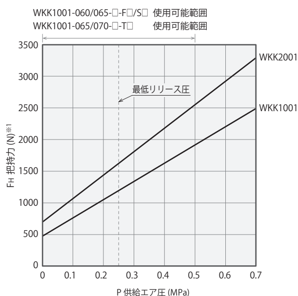
把持力線図
