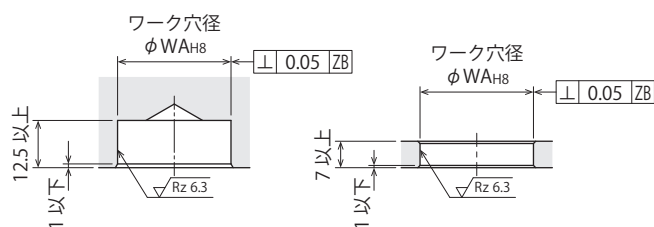
止まり穴
