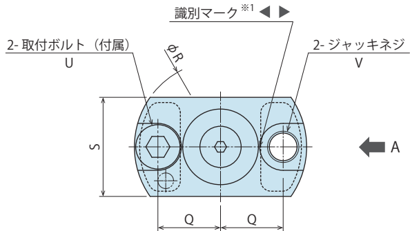
VFL-D (データム：基準位置決め用)
