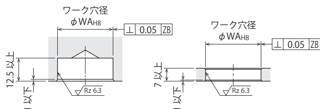
止まり穴
