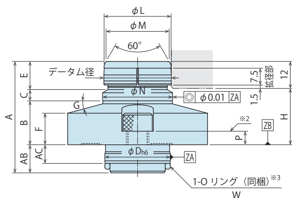
矢視 A
