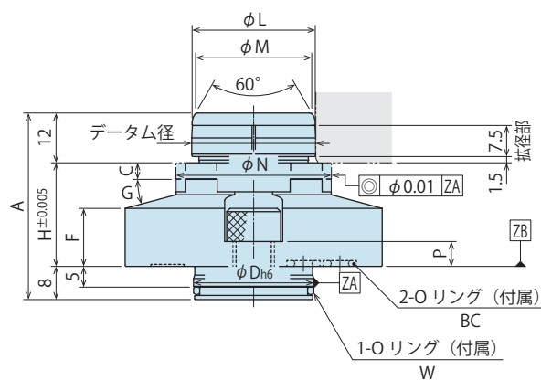
矢視 A
