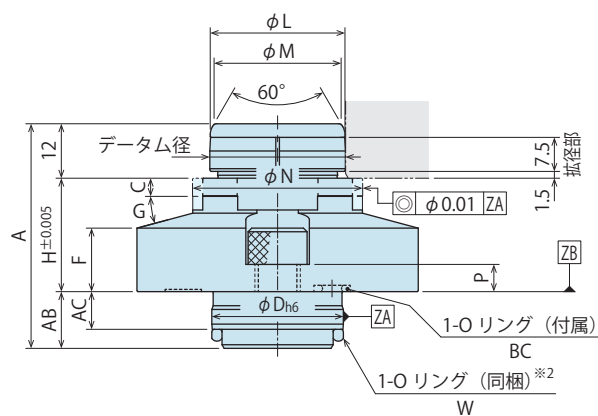
矢視 A
