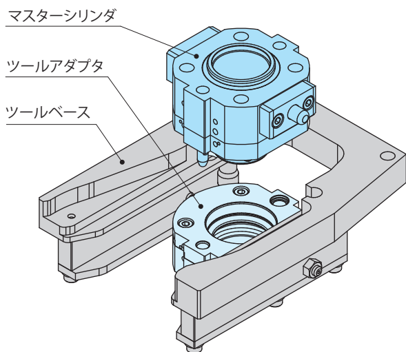
連結前の状態 (リリース状態)
