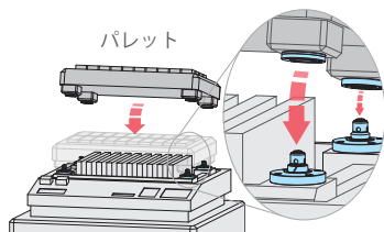
エアロケットクランプ model SWQ/SWT
