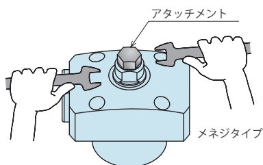
LLV□-CAE-□ / LLV□-CBE-□ : メネジタイプ
