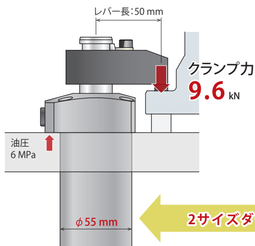
Model LHD0550 の場合
