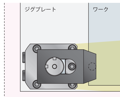
ダブルピストン油圧スイングクランプ
