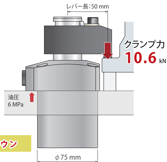
Model LHA0750 の場合
