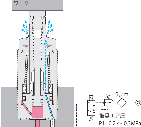
LD プランジャ上昇動作およびロック時 (エア供給入) ※1
