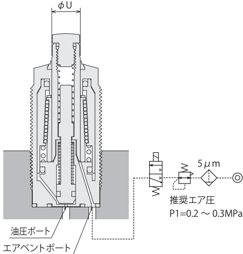
LD プランジャ下降動作およびリリース時 (エア供給切) ※1
