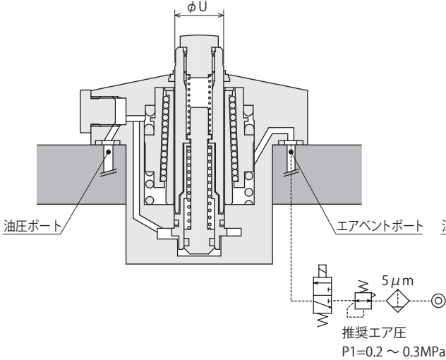
LC プランジャ下降動作およびリリース時（エア供給切）※1
