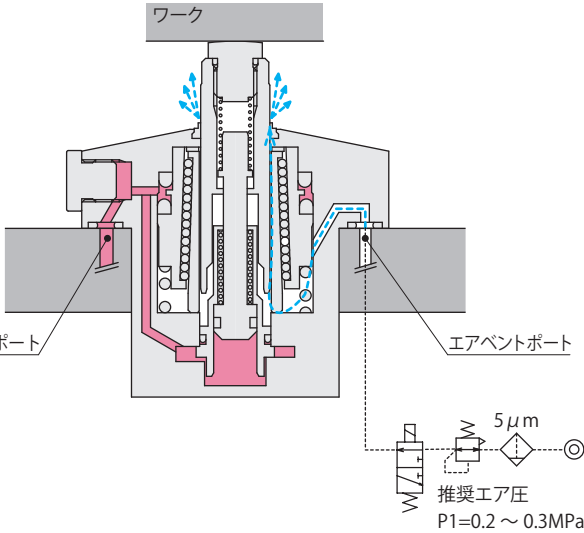
LC プランジャ上昇動作およびロック時（エア供給入）※1
