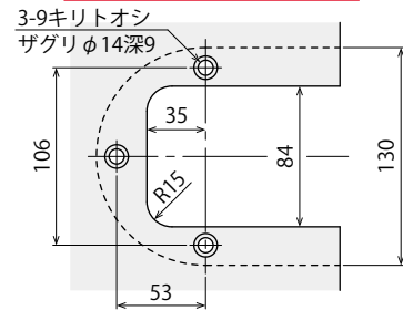
取付部加工要領 (客先殿施工)
