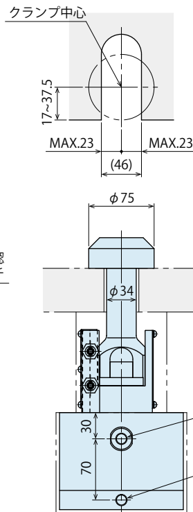
金型 U カット寸法 (客先殿施工)
