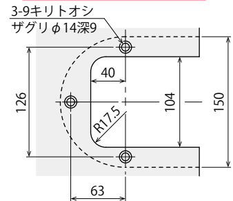
取付部加工要領 (客先殿施工)
