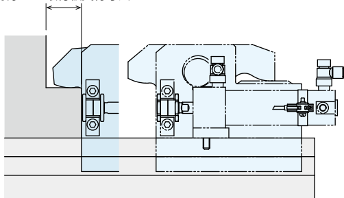
最小金型取付板奥行寸法
