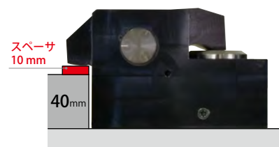
クランプ部厚さ：40mm
