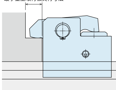
最小金型取付板奥行寸法
