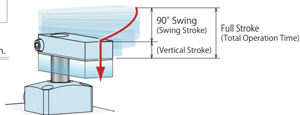
TLA0801-2
