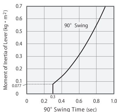
TLA4001-2
