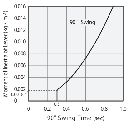
TLA1001-2
