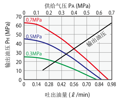
AB8000 计算公式 PH = 95(P_A - 0.04)
