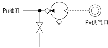
4 回路符号 无标记：标准型
