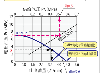
AB4000 计算公式 PH = 15(P_A - 0.04)
