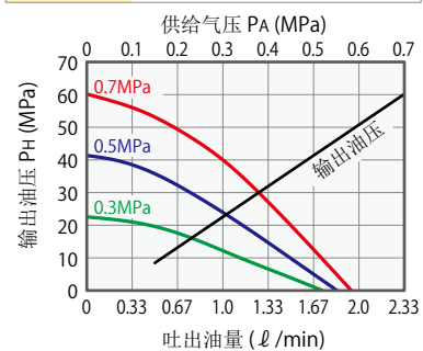
AC8001 计算公式 PH = 94(P_A - 0.06)
