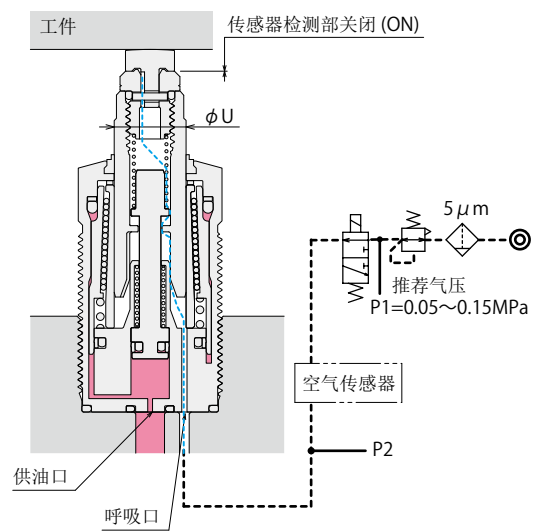
TNC 柱塞上升·工件接触 (空气传感器 ON)
