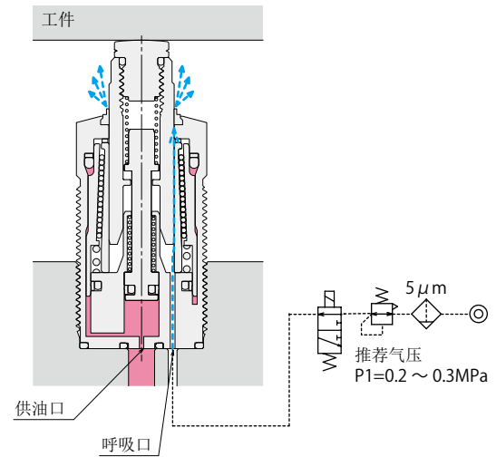
TNC 柱塞上升动作以及抱紧状态时 (供给气压) ※1
