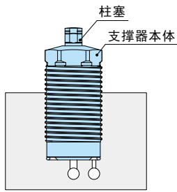
油压：OFF 上图为柱塞下降时的状态。
