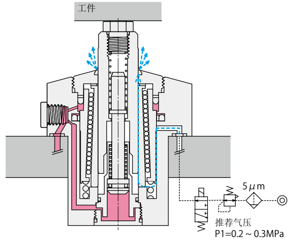
TC 柱塞上升动作以及抱紧时 (供给气压) ※1
