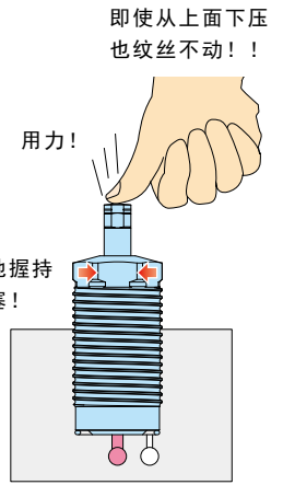
油压：ON 在供给油压作用下抱紧柱塞的动作结束，即使从上面用力往下压，柱塞也不会下降。
