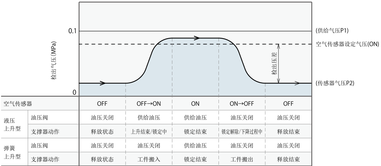
1台空气传感器连接1台支撑器 空气传感器供气压力为P1=0.1MPa时
