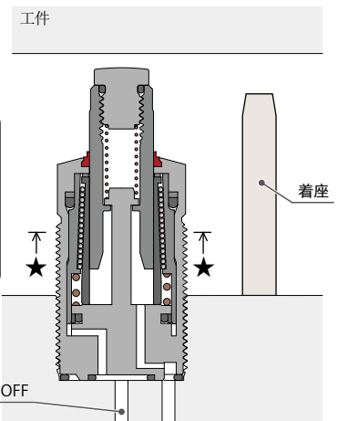
释放状态 (柱塞上升)
