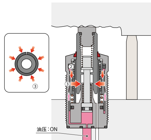
抱紧状态
