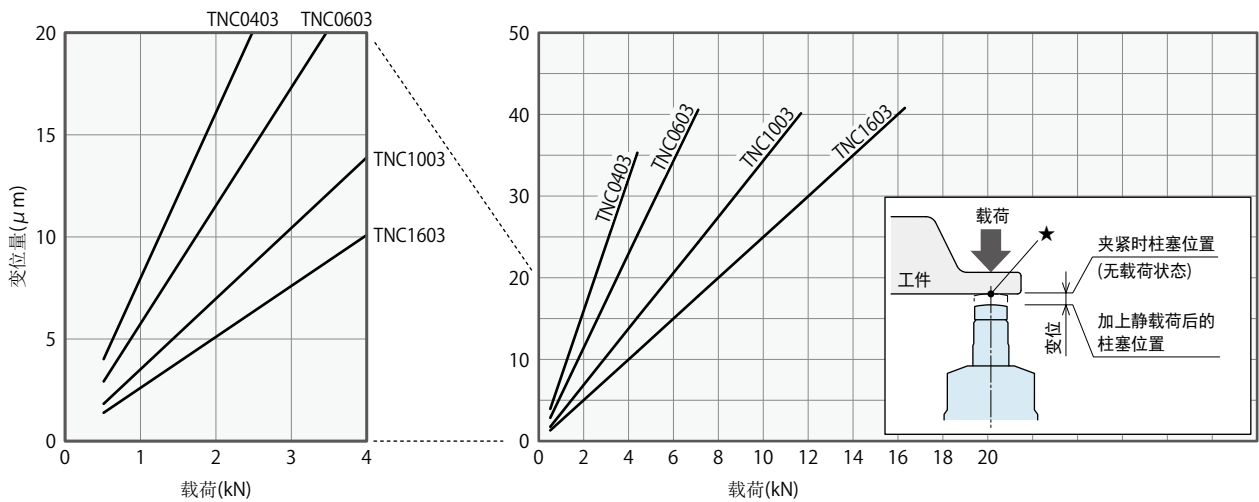
■载荷 / 变位曲线图 ★标记部位的凹凸以及因周边夹紧器等引起的工件侧变位不包含在内
