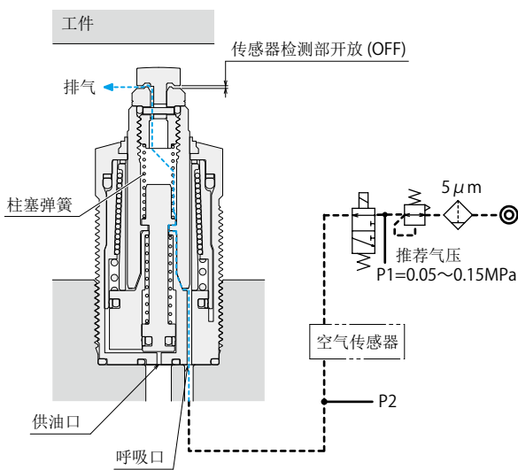
TNC 释放时 (空气传感器 OFF)
