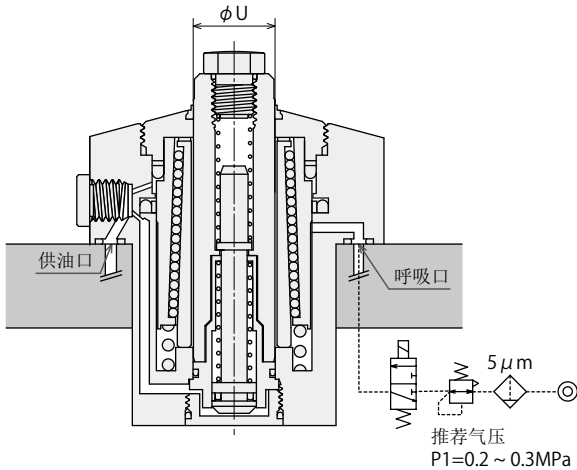
TC 柱塞下降动作以及释放时 (切断气压供给) ※1
