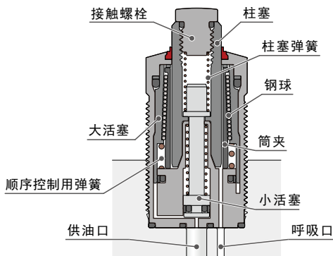
释放时 (剖面结构)
