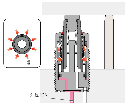
抱紧状态
