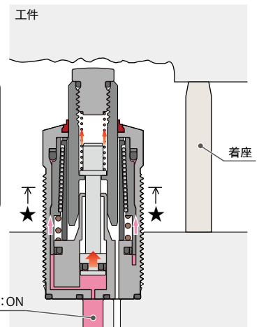
柱塞上升
