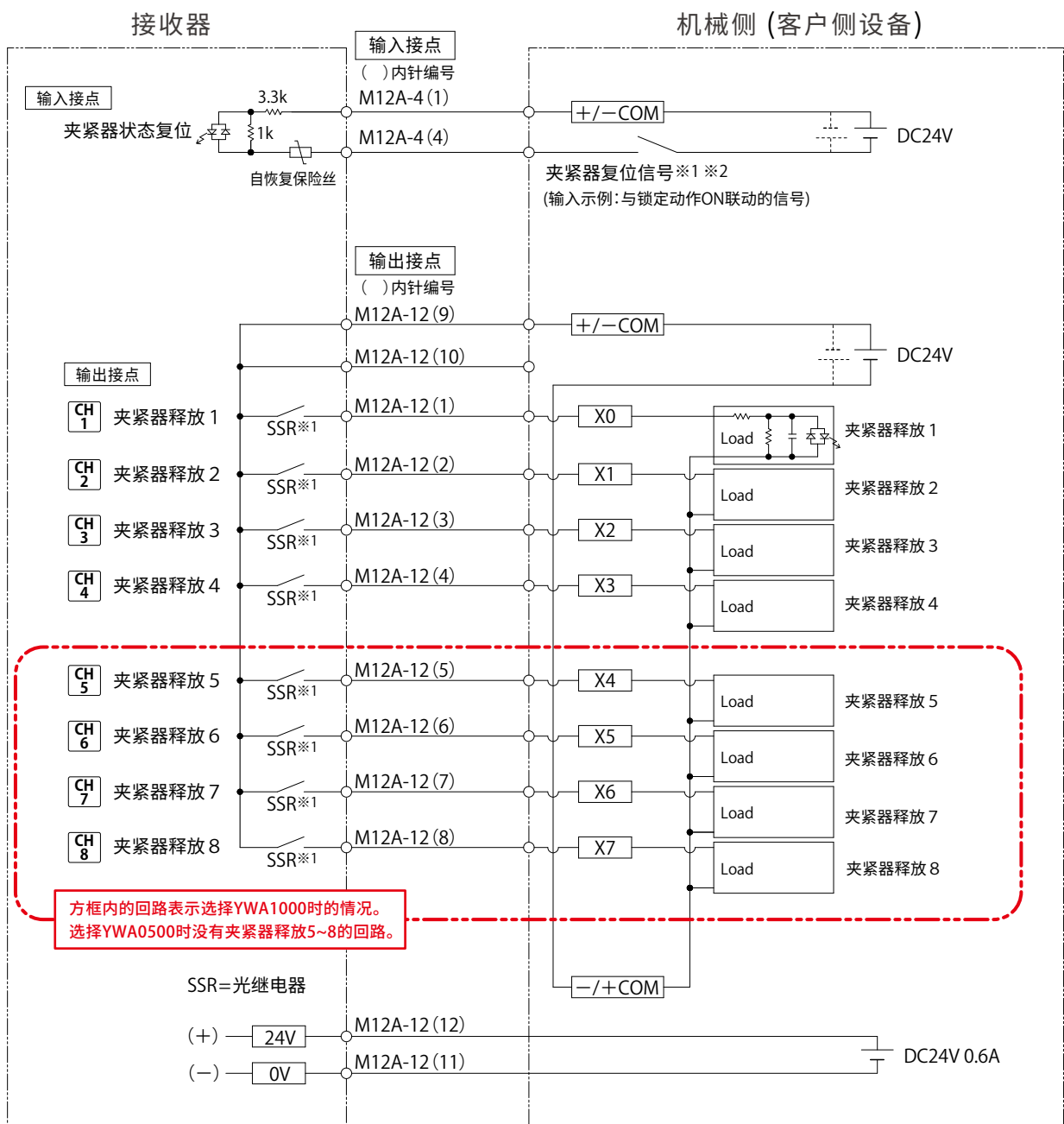
工作机器侧和接收器的接口图
