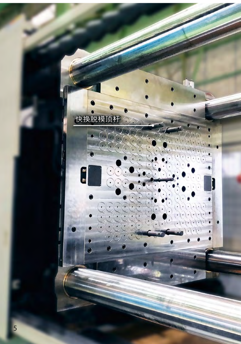
注塑机能力：1300ton 级别、电磁板：MAK1300 (板厚 50mm、控制单元数量 6、对应温度 120℃、MIMS 规格)
