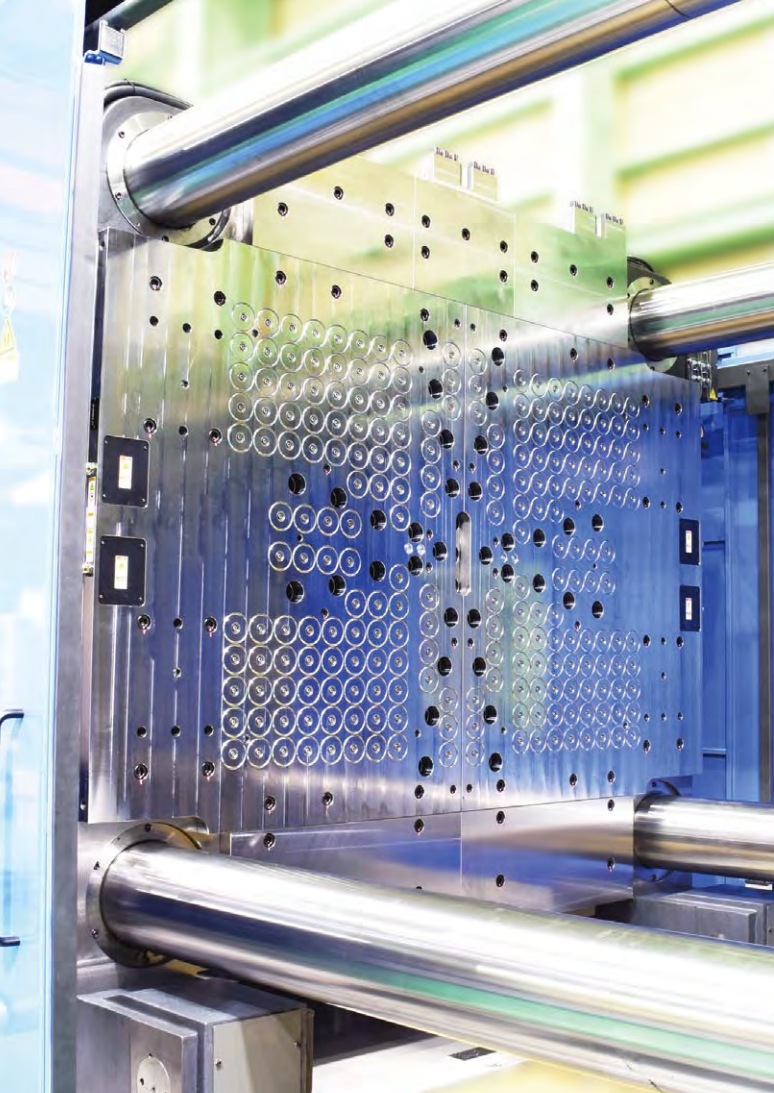
注塑机能力：1800ton 级别、电磁板：MAK1800 (板厚 50mm、控制单元数量 8、对应温度 100℃、MIMS 规格)
