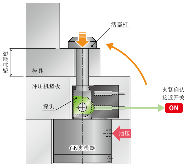
夹紧状态
