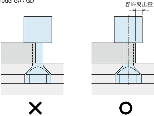
容许突出量
