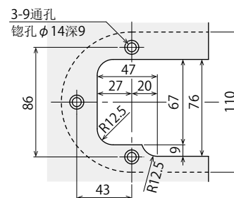
安装部加工要点 (用户施工)
