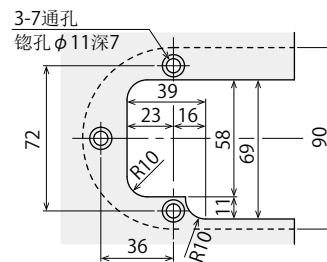
安装部加工要点 (用户施工)
