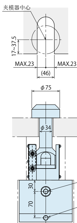
模具U形槽尺寸 (用户施工)
