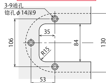
安装部加工要点 (用户施工)
