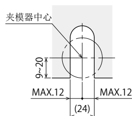
模具U形槽尺寸 (用户施工)
