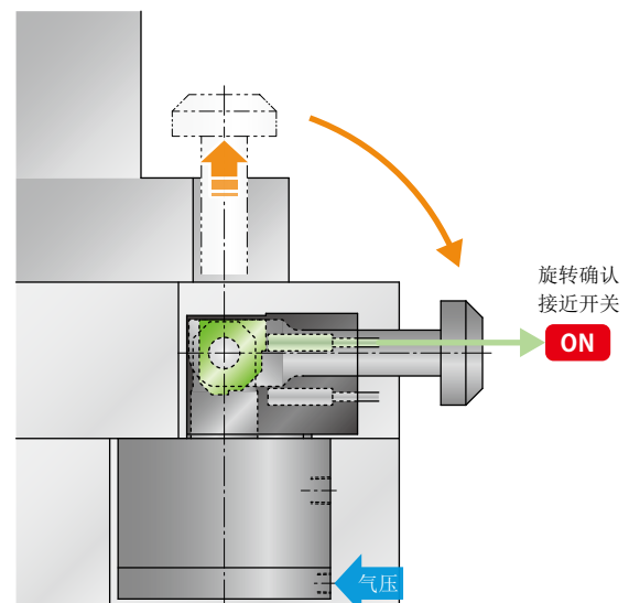
释放状态
