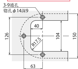
安装部加工要点 (用户施工)
