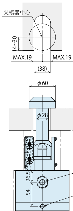
模具U形槽尺寸 (用户施工)
