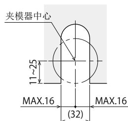
模具U形槽尺寸 (用户施工)
