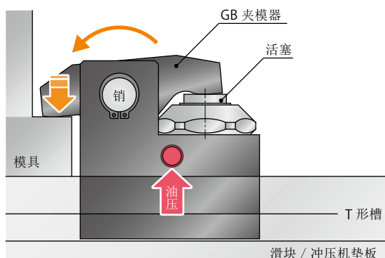
夹紧状态
