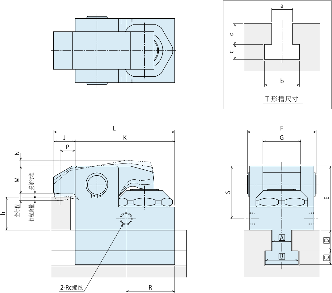
外形尺寸表
