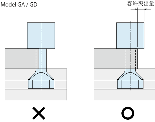
容许突出量
