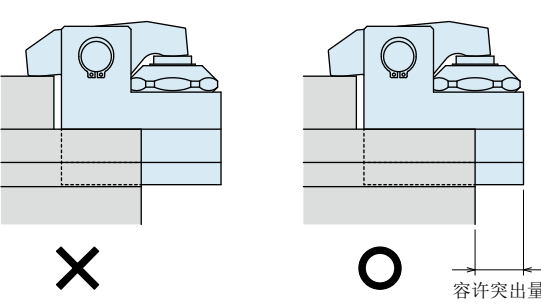
容许突出量
