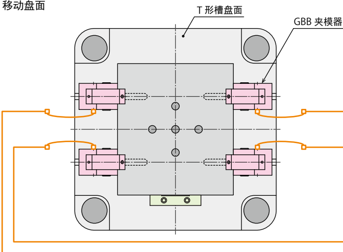
移动盘面
