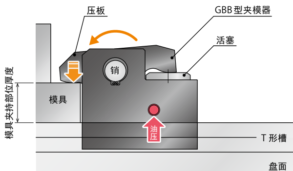
夹紧状态
