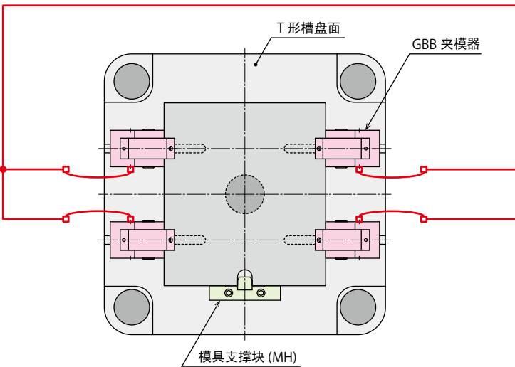
固定盘面
